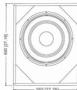
CLA-18B Subwoofer
